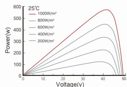
Power-voltage(570W)
